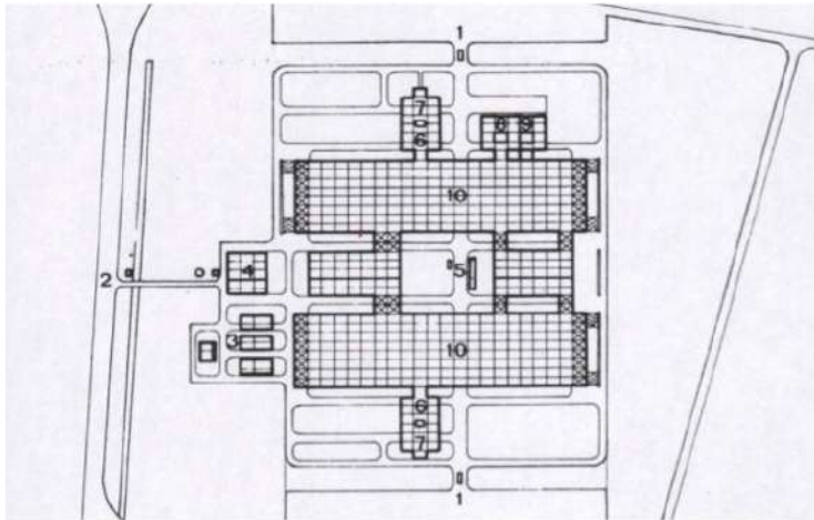
Planimetria del complesso di Marcanise.
